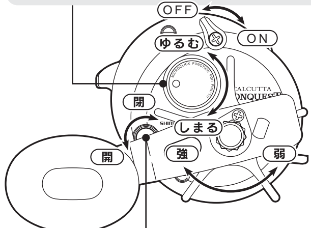
左サイドプレート開閉つまみ
